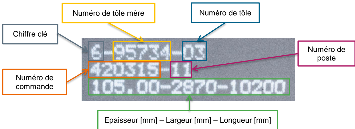
Figure 2: marquage peinture standard DH (aperçu)
