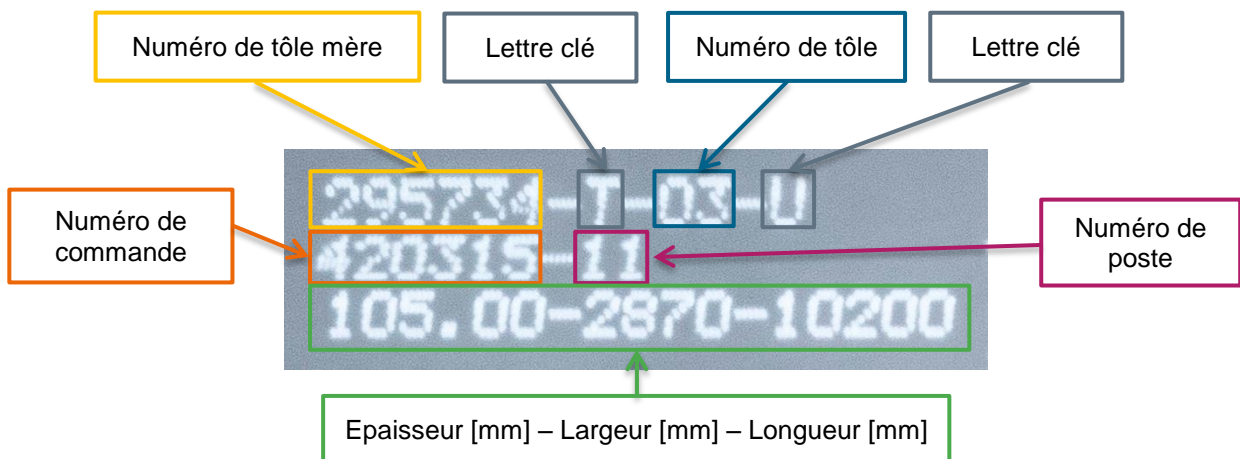
Figure 3: marquage peinture standard DF (aperçu)
