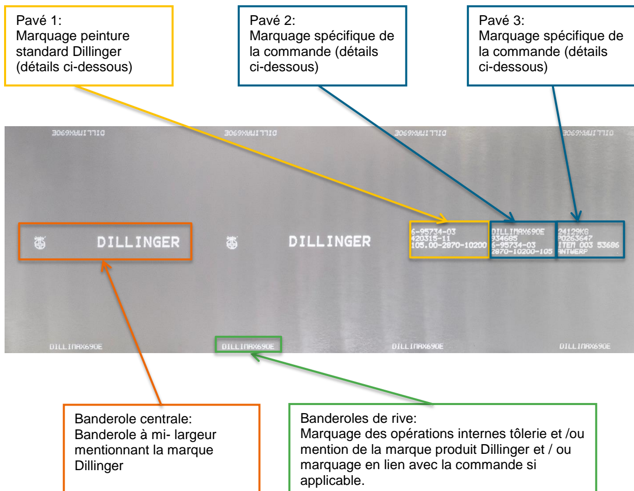
Figure 1: Structure du marquage peinture Dillinger (aperçu)
